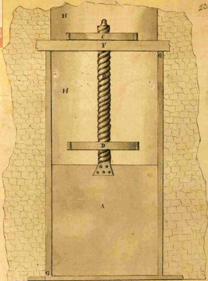
Compuerta de Tornillo.
